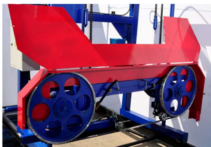
Рабочие габариты станка
